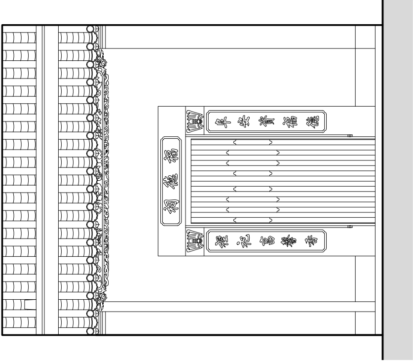
正立面圖 ALÇADO
