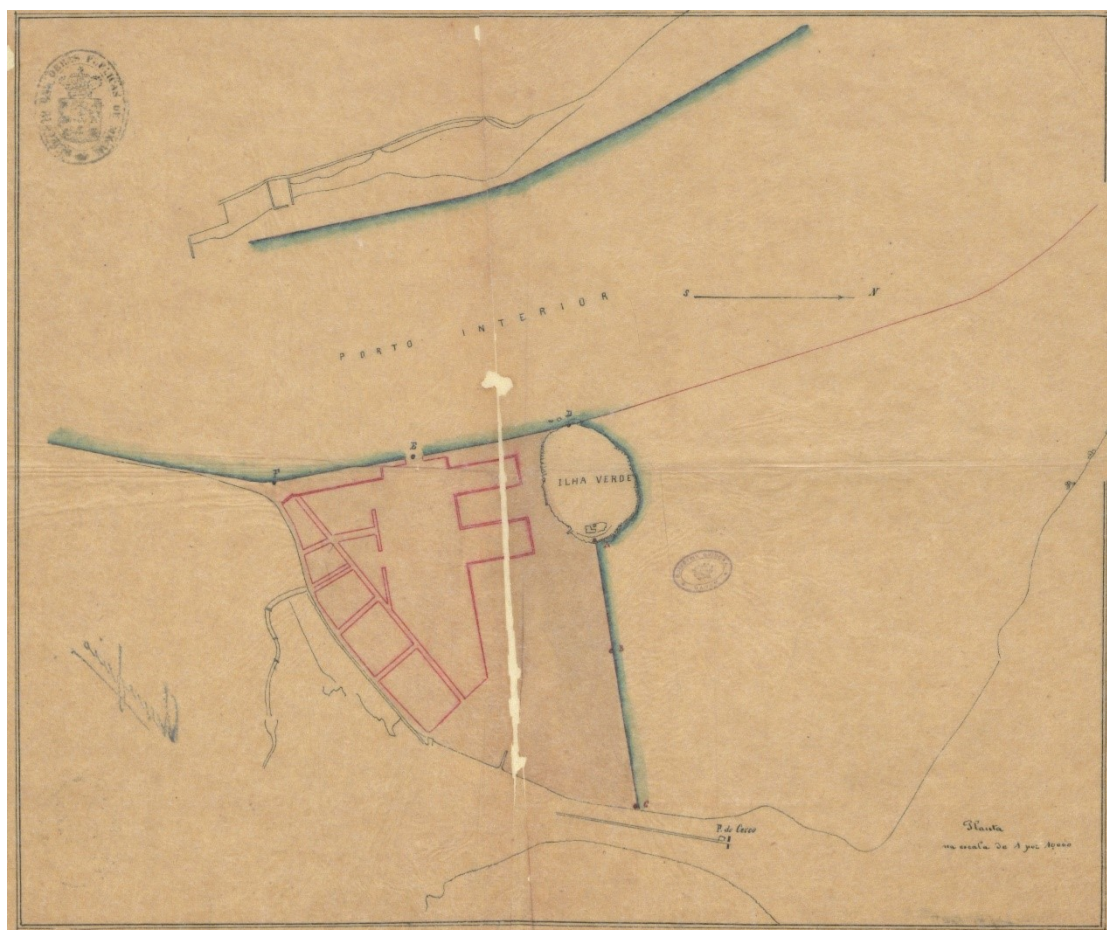
1887 年青洲與林茂塘之間海灣的填海計劃，並有意在此建造避風塘。
