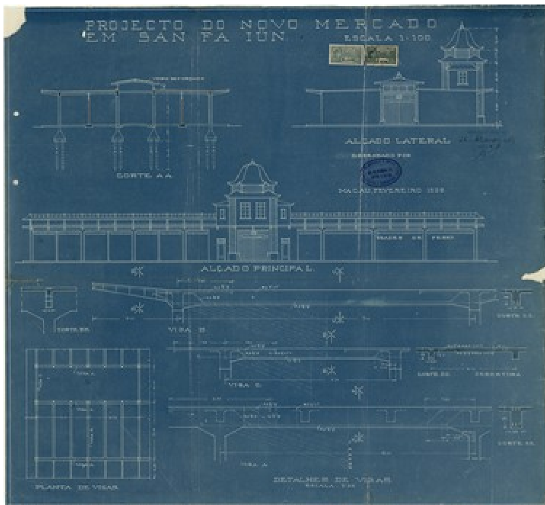
1928 年由利味調及米路畫則工程師設計的下環街市建築方案，以現代鋼筋混凝土結構，而入口塔樓與側立面帶中國式的風格。
