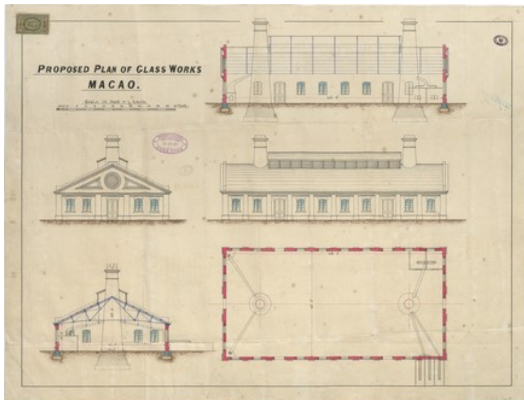
1884 年丹比與利公司的澳門玻璃廠計劃圖，採用西式古典設計，坡屋頂採用金屬桁架支撐，並建有兩個大煙窗。
