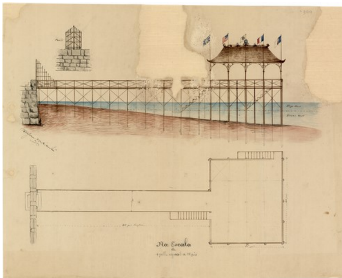
約 1905 年桔仔街前地的建造碼頭計劃，碼頭以椿柱建於堤岸邊，並建有中式屋頂的亭。
