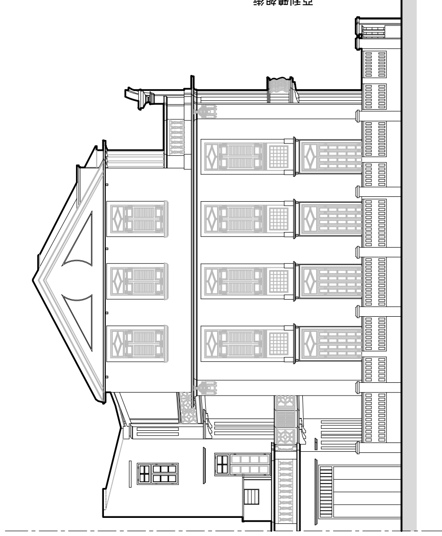
側立面圖 ALÇADO
